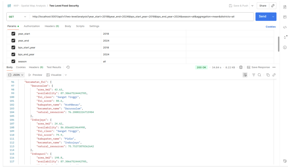
Gambar 4.15. Analisis FSI dari backend Flask
